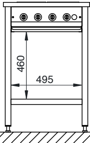
FST/FSTH 4090
