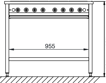
FST/FSTH 8090
